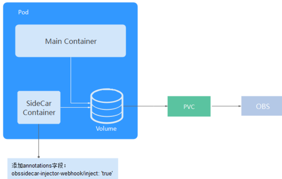
图 8-11 SideCar Container
